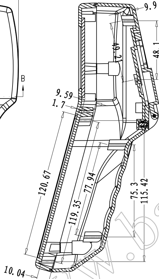
SEC A-A
